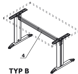
TYP B BELKA STALOWA w kształcie rynny, służąca do przeprowadzenia okablowania
