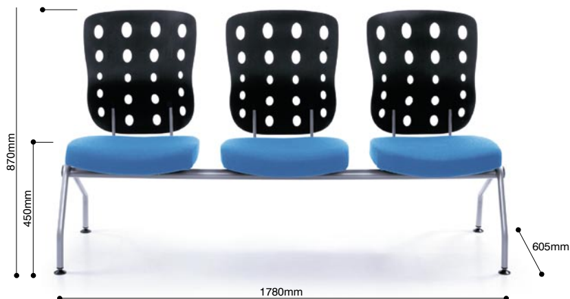
UWU 20 L3 29 kg brutto D / W / H 670 / 1790 / 900 mm
