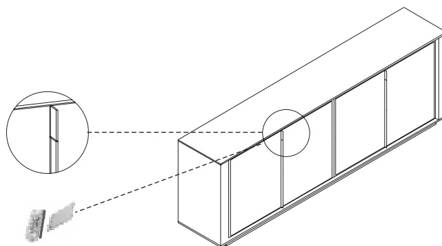
UCHWYT Z ALUMINIUM ANODOWANEGO ZAMEK NA KARTĘ
