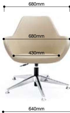
FAN 10 E
